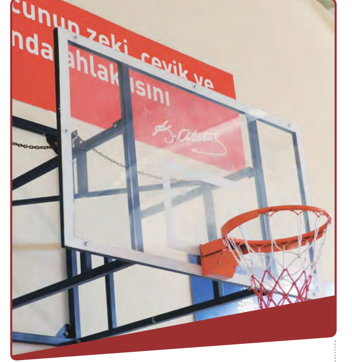
Basketbol Potası Duvara Montaj Yana Katlanabilir 10 mm Cam (Ak) Panya 105 x 180 cm 20 Sabit Çember
