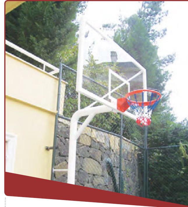
Basketbol Potası, Tek Direk Boru (4"114/4,5mm) 15 mm Cam (Ak) Panya 105x180 cm 20 Sabit Çember
