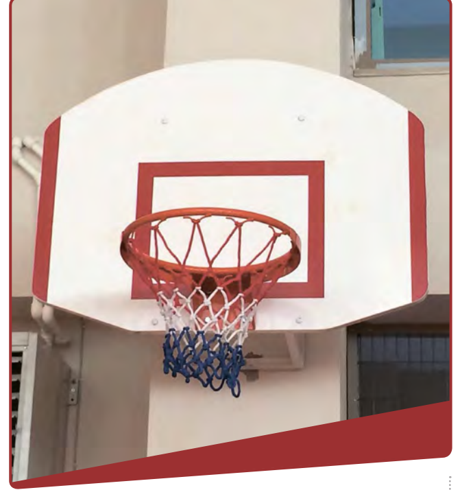
Basketbol Potası Duvara Montaj Antrenman Fiber Amerikan Panya 90x120 cm 20 Sabit Çember
